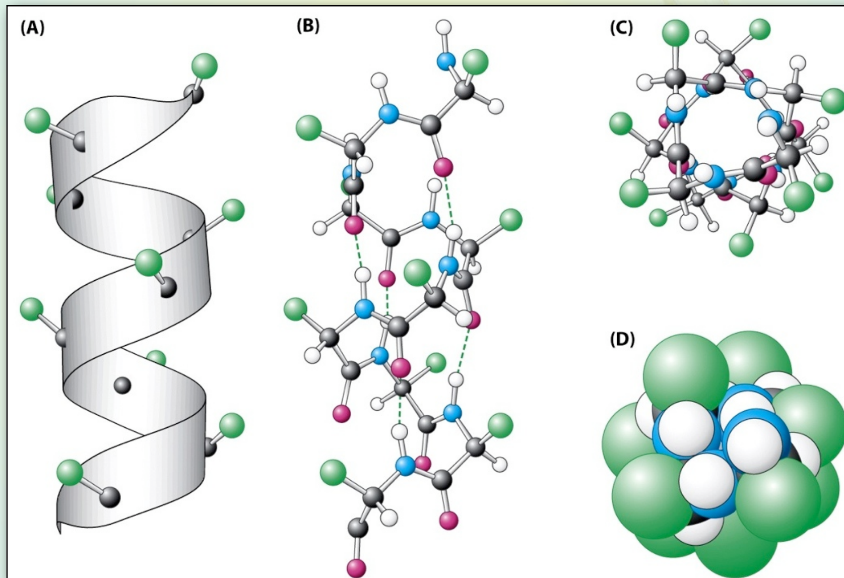
\alpha -helix
