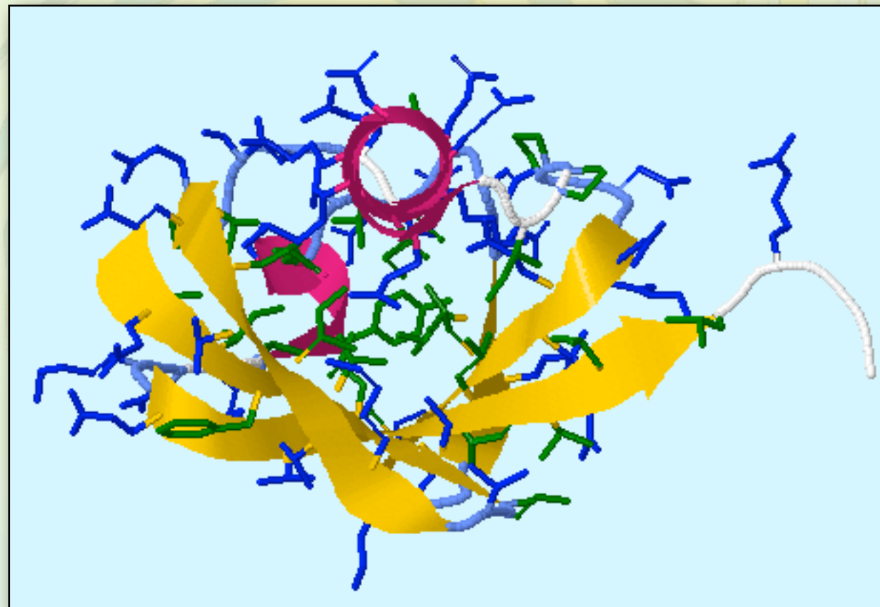
Ubiquitin
