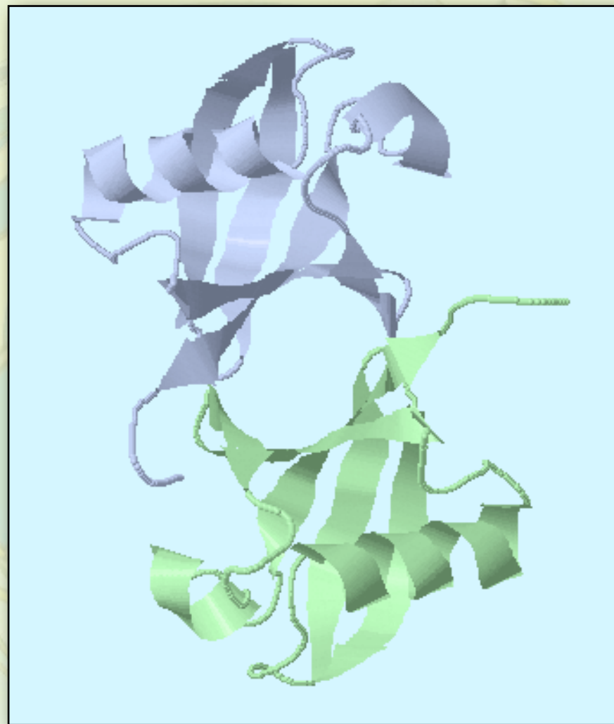
Ubiquitin
