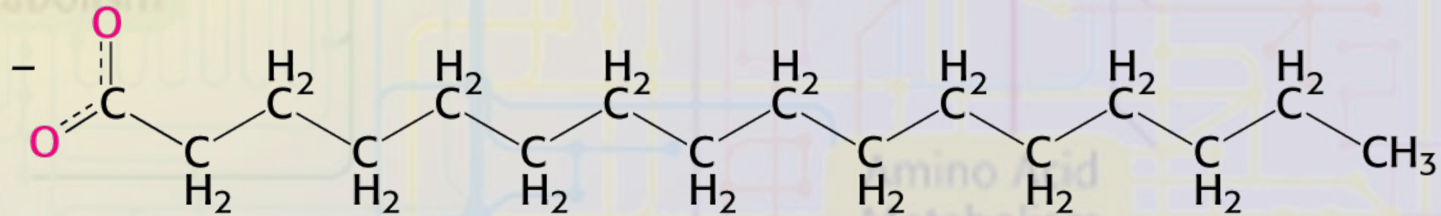
Fatty acid
